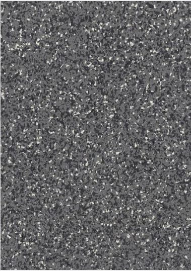
Materia oscura
